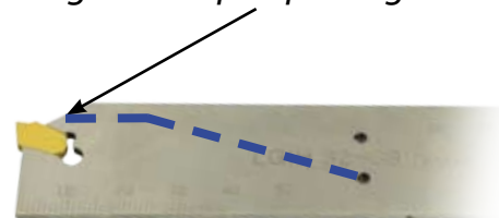
Chłodzenie podawane na płytkę Cooling to the tip of parting-off insert
